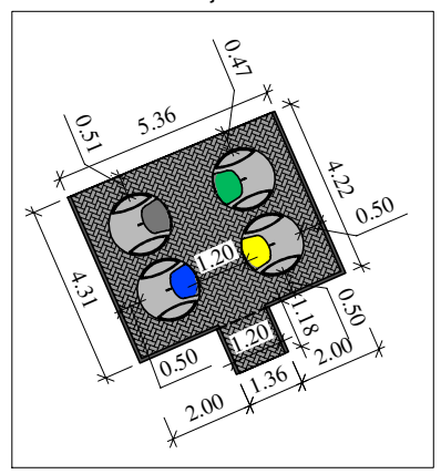
Aikštelės detalizacija
