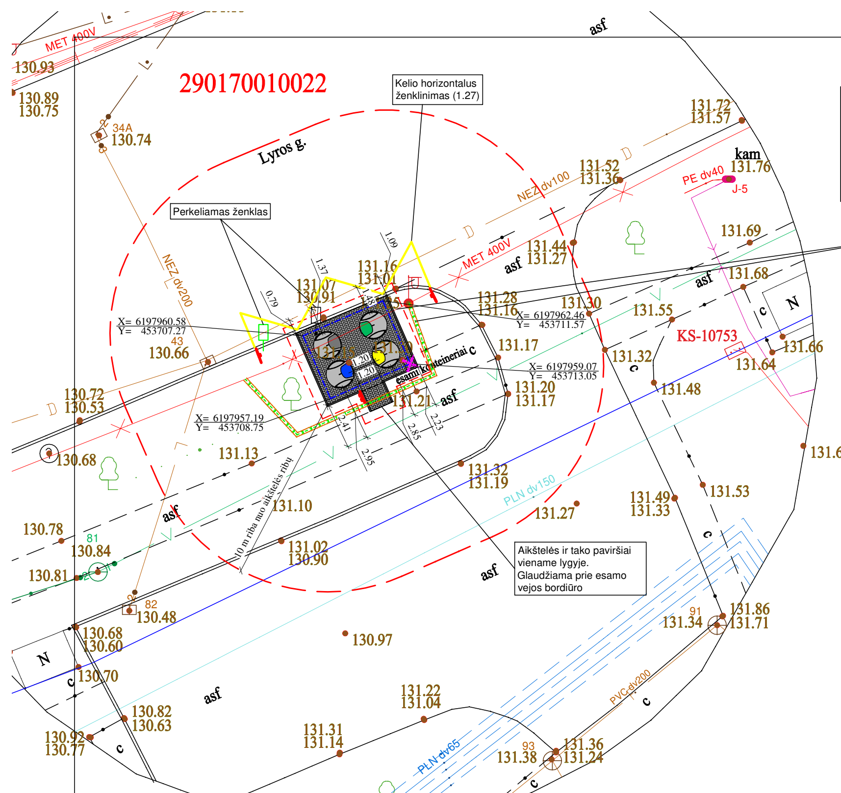
Aikštelės detalizacija
